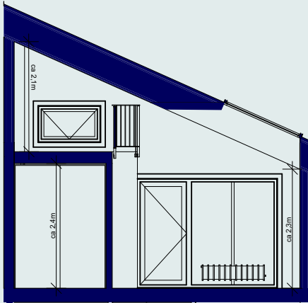
Snitt A-A
