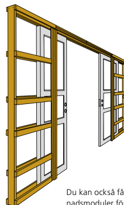
Tvärsnitt av skjutdörrs-parti för enkeldörr.
